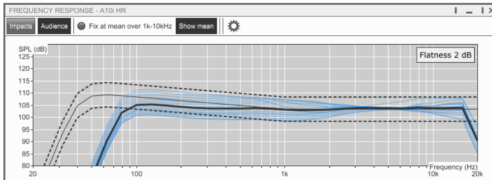
Figur 3 Frekvensrespons
