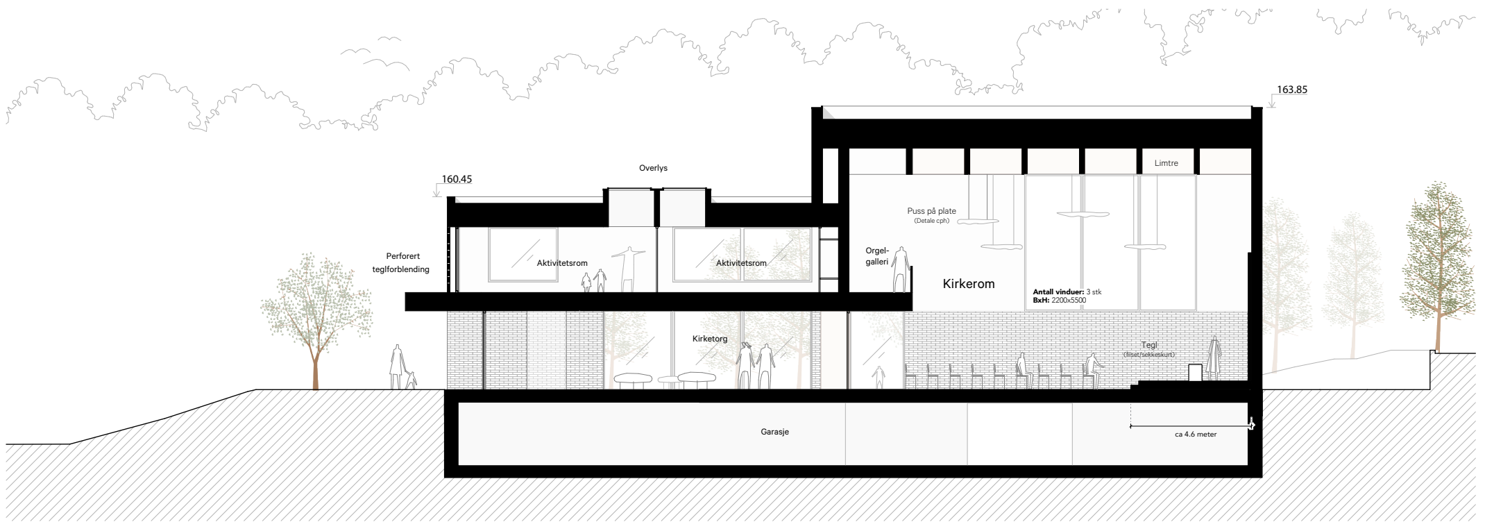
Snitt B
