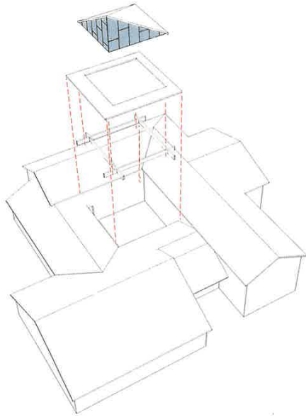
EKSPLODERT DIAGRAM KONSTRUKSJONSPRINSIPP
