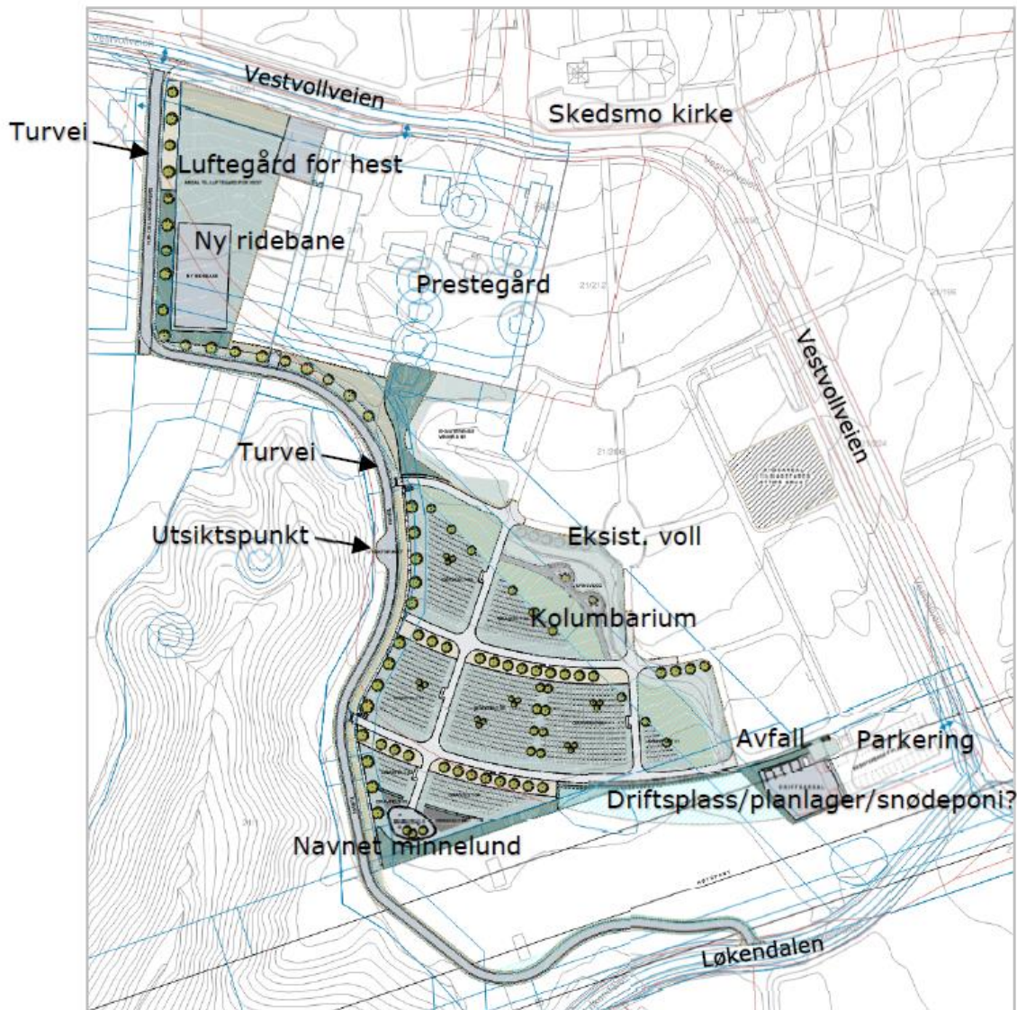
Utsnitt av gravplassplanen, tegning 10-700-00-202 (ill. COWI/Arkitema)
