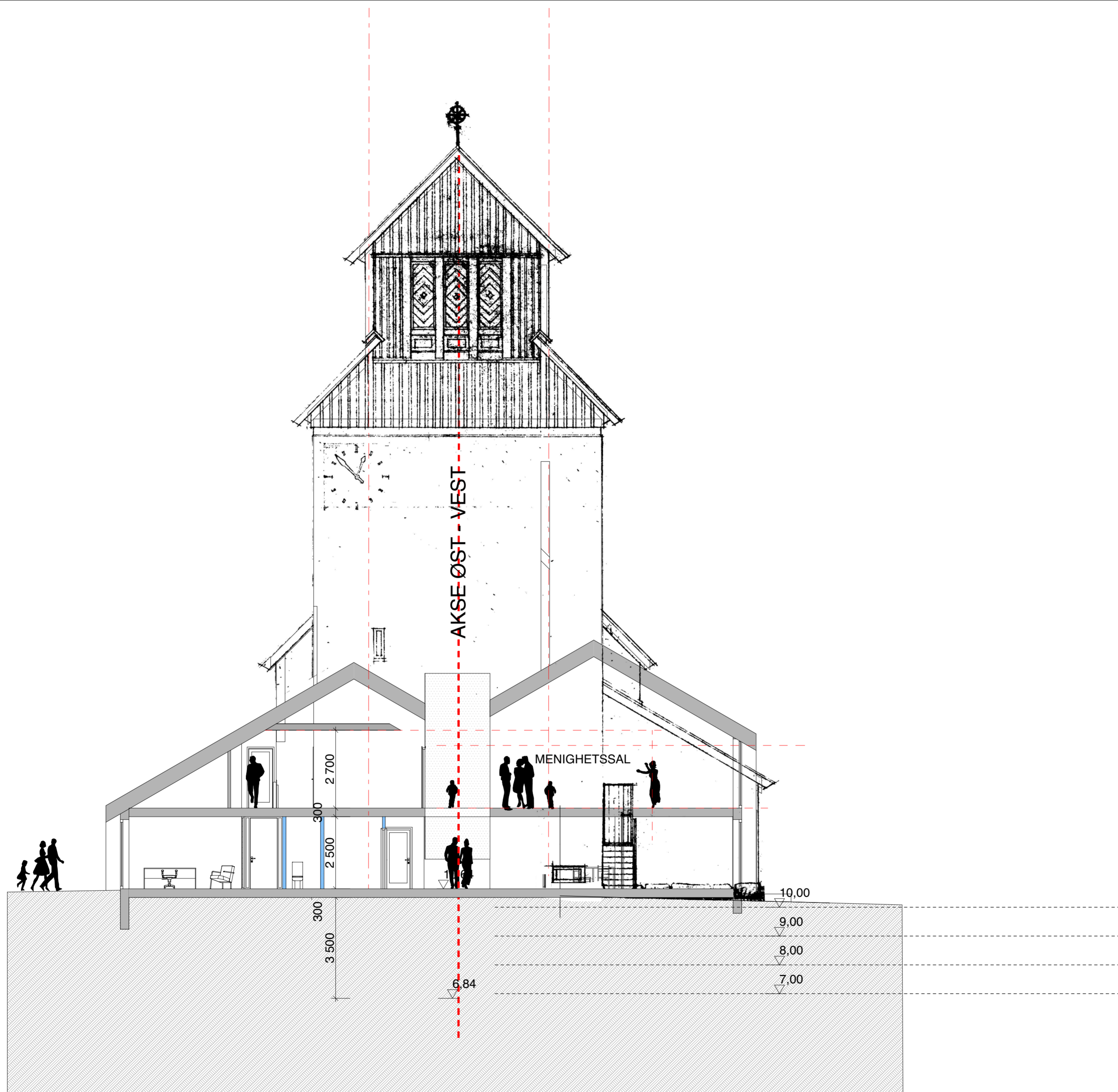
1:100 Snitt A
