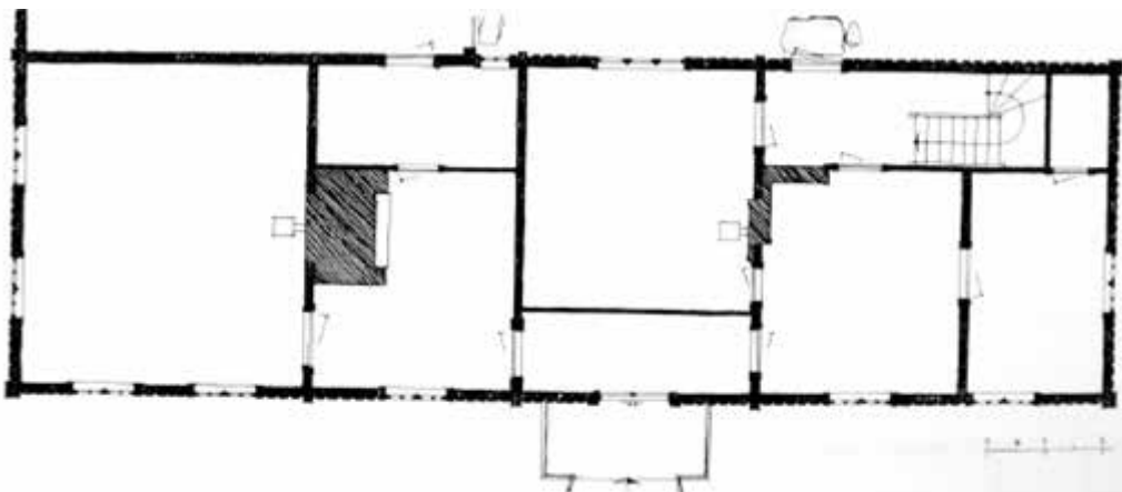
Hovedbygningen, plan over første etasje.
